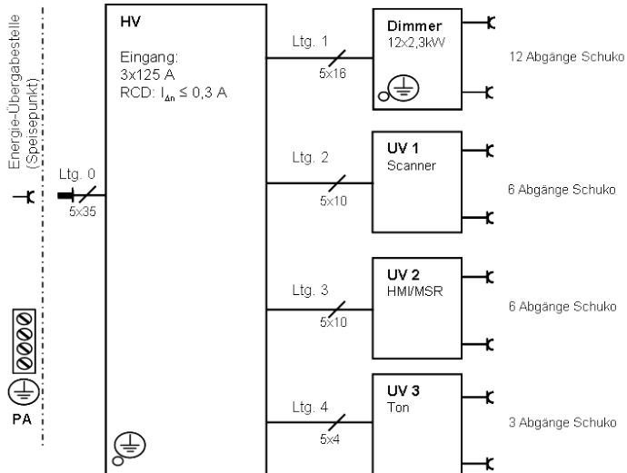
Abb. 7: Übersichtsplan – Energieversorgung für eine kleine Veranstaltung
