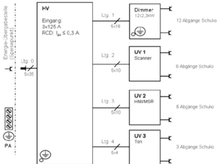
Abb. 7: Übersichtsschaltplan – Energieversorgung für eine kleine Veranstaltung
