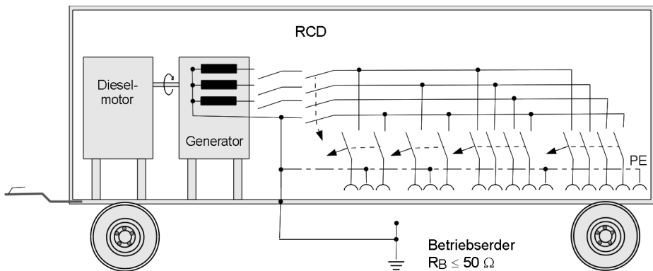
Abb. 2: Stromerzeuger im TN-S-Betrieb
