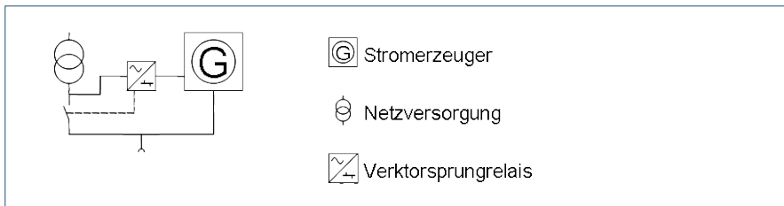
Abb. 5: Umschaltung Netz – Stromerzeuger mittels Vektorsprungrelais
