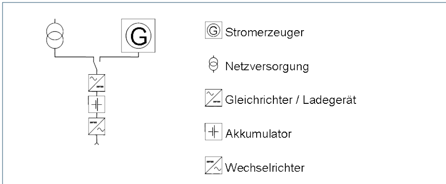
Abb. 4: USV – Anlage mit Stromerzeugerbetrieb
